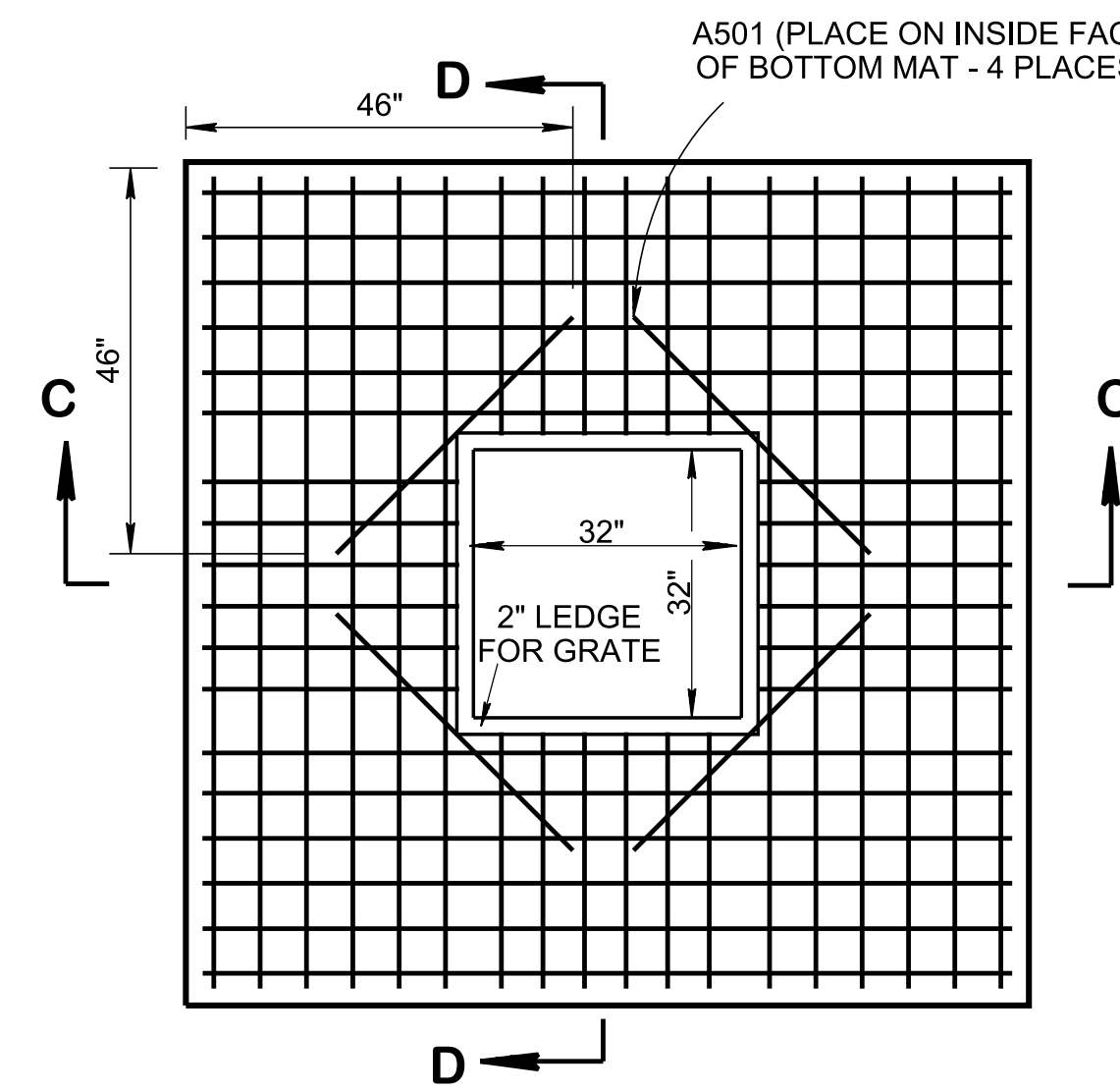
LID REINFORCING
