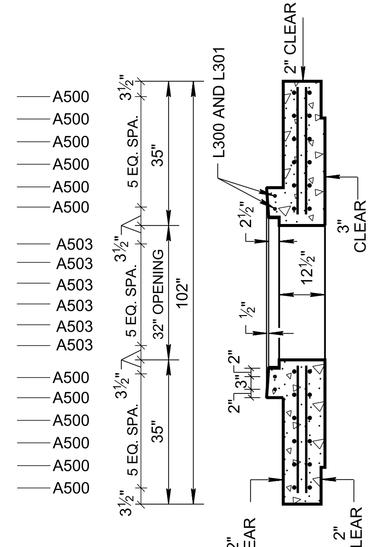
SECTION D-D
