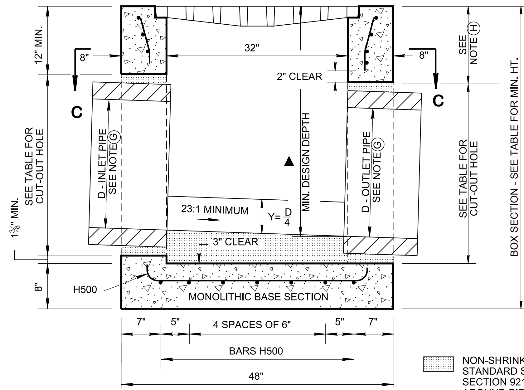
SECTION A-A
