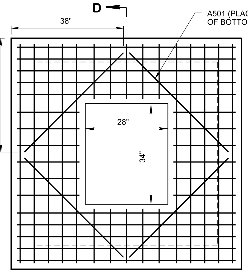
LID REINFORCING
