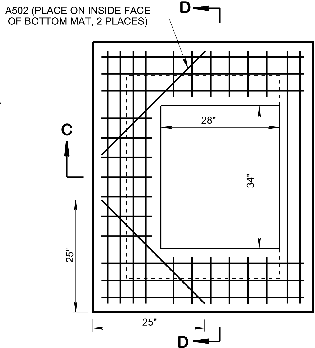
LID REINFORCING
