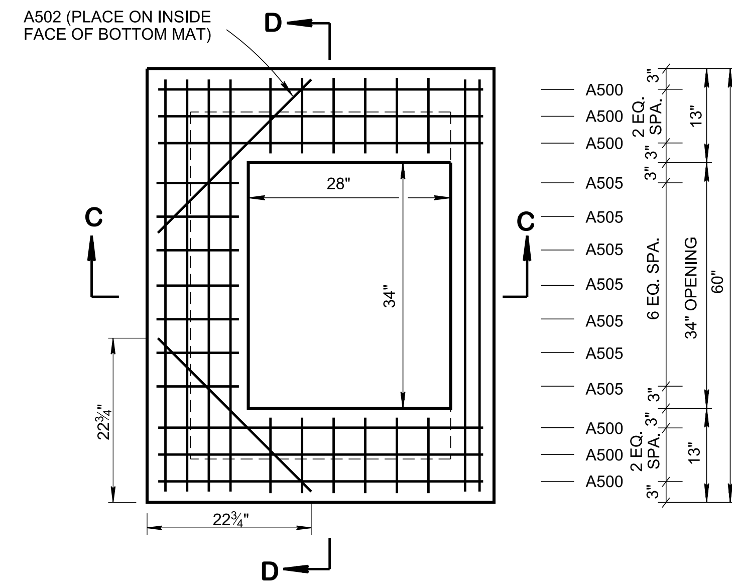
LID REINFORCING
