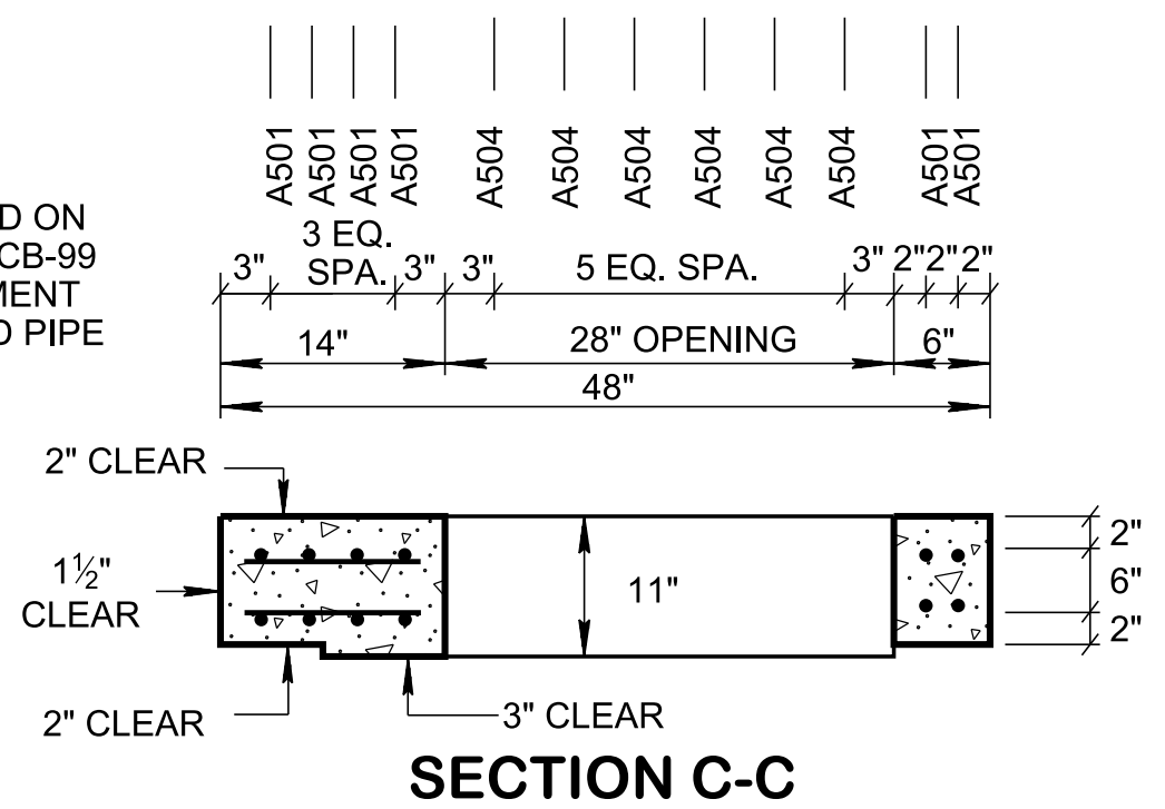
LID REINFORCING
