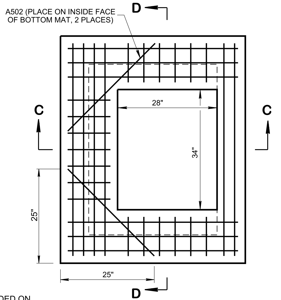
LID REINFORCING
