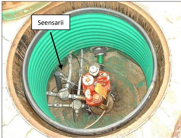
Saampii taankarii kan agarsiisu gaaskitii golgaa saampii bakka isaa fi sensor bakka sirrii ta'e qabsiisuu
