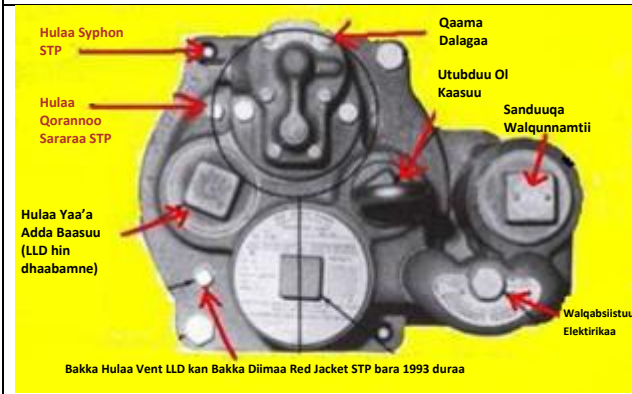
Paampii bishaan keessaa FE Petro (hulaa taankarii jalaa) irratti tuubii qilleensaa MLLD sirritti dhaabuu.
