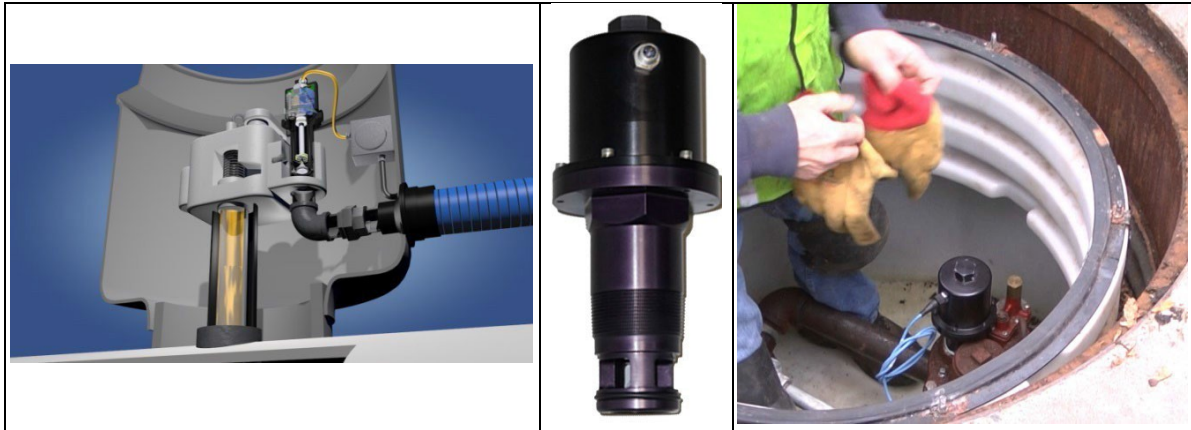
دۆزەرمووی دزەکردنی ھێلی (OPW Model 327) جوۆری قەبارمیی (VLLD)
