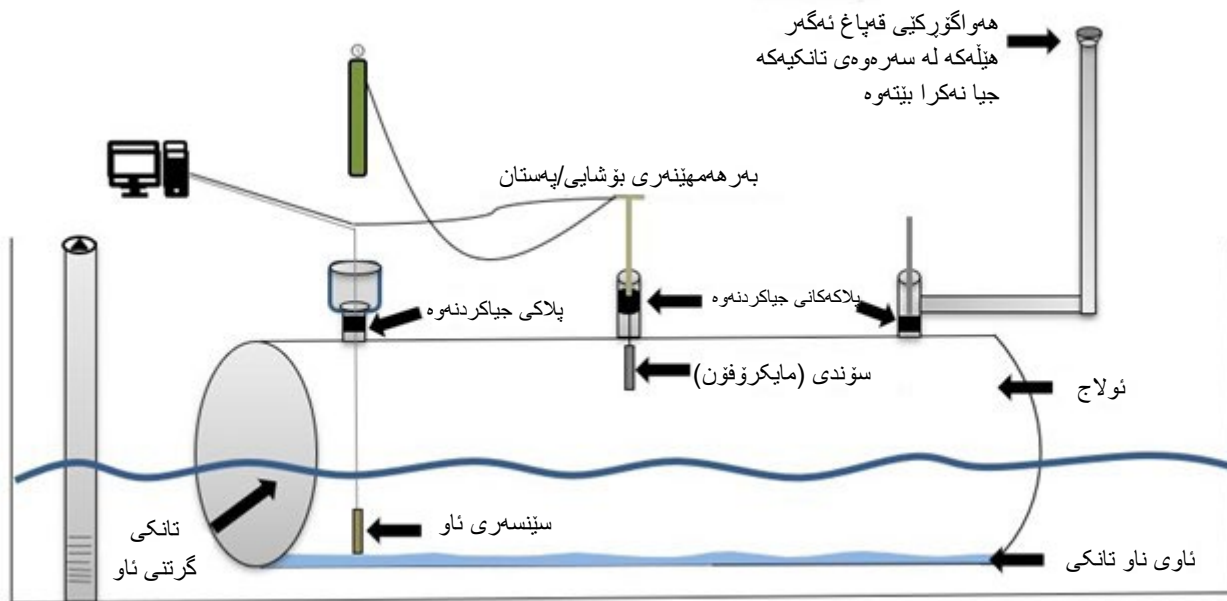
شیوهی 5. سینتهپی تاقیکردنهمهوهی بهتال یان نولاج لهگهل تانکی گرتتی ناو کهوا بهرکهوتتی لهگهل بهشهی دهرهکی تانکی هیه بهکار هینانی سینسهری ناوی شیواز مکه پیویسته.
