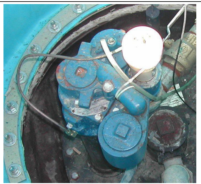
بەستانی دروستی تیوبی ھەواگۆرکینی MLLD لە سەر پەمپی غەمبەسی FE Petro (پۆرتی خوارەوی تانکی)
