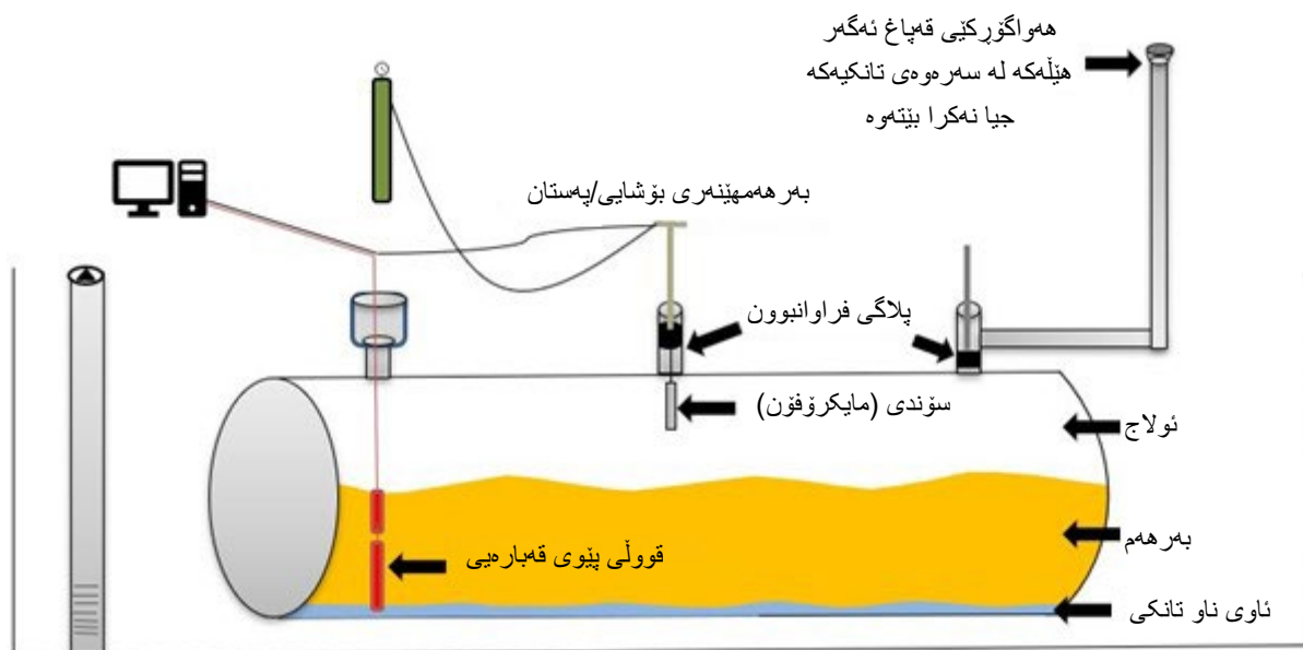
شئیوهی 1. تاقیکردنهوهی تانکی قهبارهی گشتی
