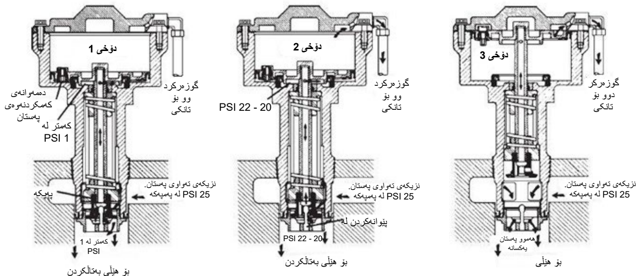
هێلکار یەكەى سەرەوه سى دۆخى شیوازی پستۆنى نمونەى MLLD نیشان دەدات
