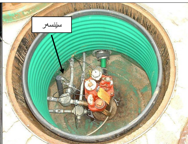
حموزی تانکی کهوا گاسکیتی قهباغی تانکی و سنسور له دۆخی دروستی نیشان دهدات
