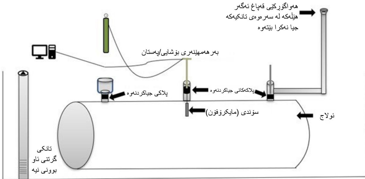
شېۋە 7. سېتەپى تاقىكردئەو بەتال يان نولاج بىن تانكى گرتتى ئاۋ كە بەر كەوتتى لەگەل بەشى دەرەكى تانكى ھەبېت سېنسىرى ئاۋ پېۋىست نىە.
