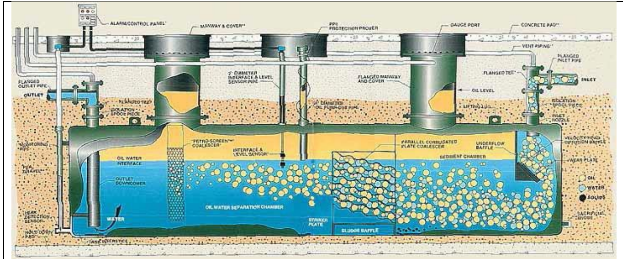
نهم شنیو به بندکردنهی خوار موه تانکیه کی ریخراو نیشان دهدات - تانکی هملگرتنی B
