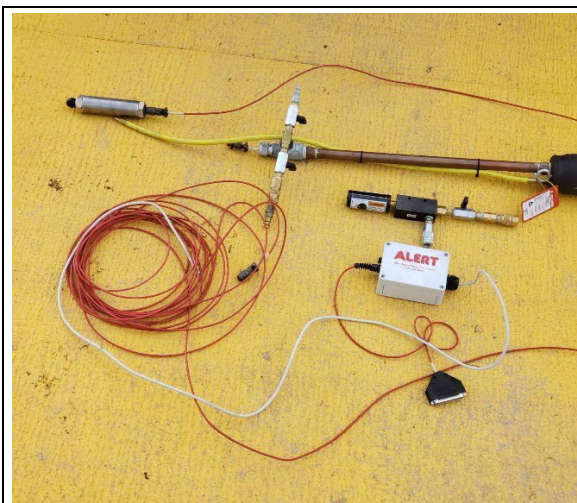
نامرازی تاقیکردنهوهی نولاجی ناگادار کردنهوهی 8200 (بهشی بهتالی تانکی) له پلاگی فراوانیون، بهر هممهینهری بوشایی/پهستان و مایکروفون پینگ دیت.
