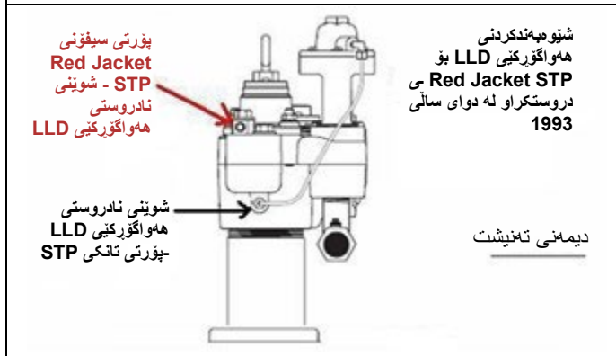
بەستانی نادروستی تیوبی ھەواگۆرکینی LLD ھەواگۆرکینی LLD ی بۆ پۆرتی سیفۆنی پۆرتی ھەواگۆرکینی تانکی STP، بەستانی نادروستی تیوبی ھەواگۆرکینی LLD
