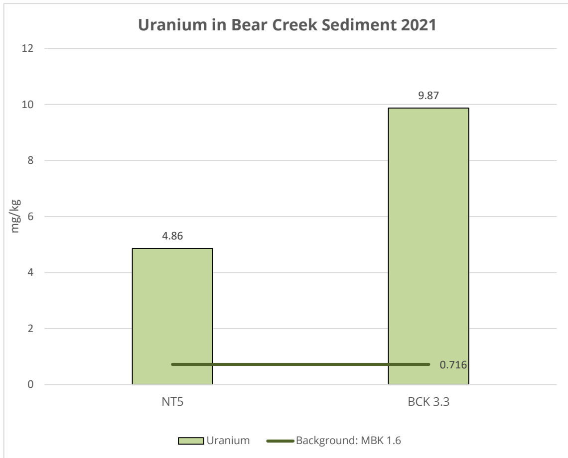
Figure 10.1.9: Sediment Uranium
