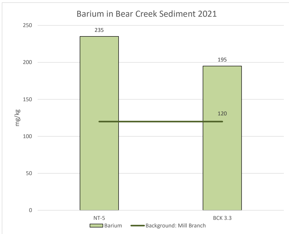
Figure 10.1.2: Sediment Barium
