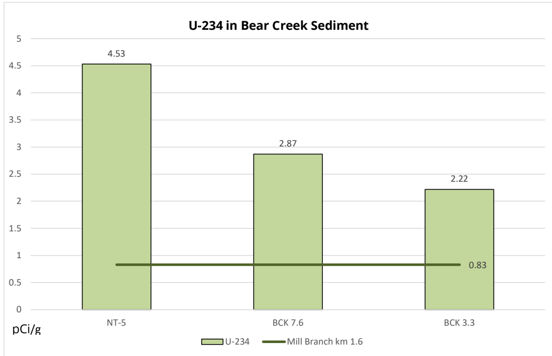
Figure 10.1.12: Sediment U-234
