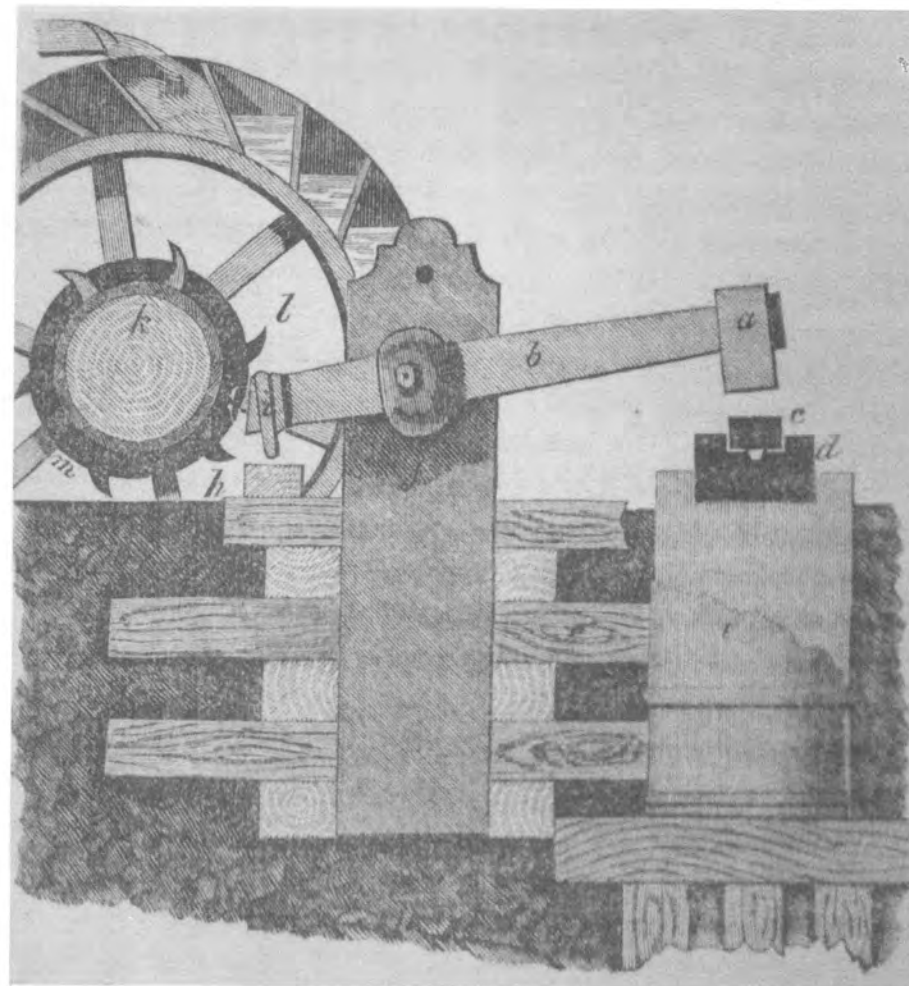
Tilt hammer.
